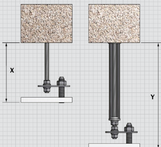
Montagebeispiele bei abgehängten Decken
